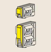
Campana de protección anti nieve izquierda de acero inoxidable Ref. RAS-(2.0-3.0)WHVRP1 y RASM-(2-3)VRE: - ASG-SP10LTBS (semi) Precio: 225 € Ref. RAS-(4.0-10.0)WH(V)NPE y RASM-(3-6)(V)NE: - ASG-NP280LS4 (semi) Precio: 370 € - ASG-SP11LAS2 (completa) Precio: 370 €
