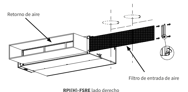
RPI(H)-FSRE lado derecho
