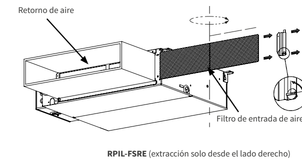
RPI(L)-FSRE (extracción solo desde el lado derecho)
