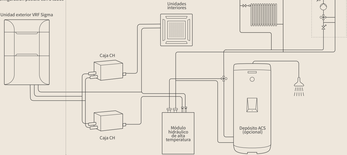
Ejemplo de configuración posible con 3 tubos
