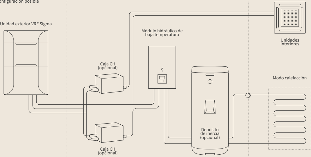
Ejemplo de configuración posible
