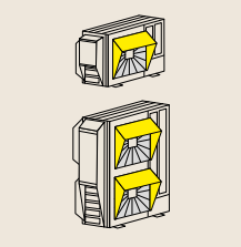
Campana de protección anti nieve frontal de acero inoxidable Ref. RAS-(2.0-3.0)WHVRP1 y RASM-(2-3)VRE: - ASG-SP10FTBS (semi) Precio: 275 € - ASG-SP11FTBS (completa) Precio: 370 € Ref. RAS-(4.0-10.0)WH(V)NPE y RASM-(3-6)(V)NE: - ASG-NP335FS4 (semi) Precio: 250 € - ASG-SP11FCS2 (completa) Precio: 400 €
