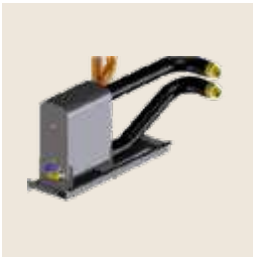
Recuperación parcial de calor 50 % Intercambiador de placas adicional, instalado en la descarga del compresor, delante de los intercambiadores de calor de aire. Ref.: PHR50
