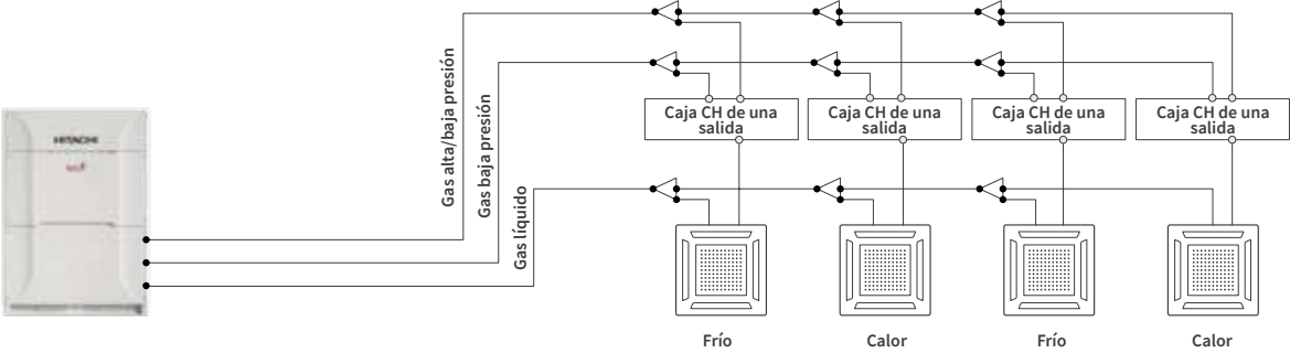
Caja CH de una salida: conexión en 2 tubos (solo líneas de gas)
