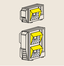
Campana de protección anti nieve frontal de zinc Ref. RAS-(2.0-3.0)WHVRP1 y RASM-(2-3)VRE: - ASG-SP10FTB (semi) Precio: 320 € - ASG-SP11FTB (completa) Precio: 375 € Ref. RAS-(4.0-10.0)WH(V)NPE y RASM-(3-6)(V)NE: - ASG-NP335F1 (semi) Precio: 330 € - ASG-SP11FC (completa) Precio: 850 €
