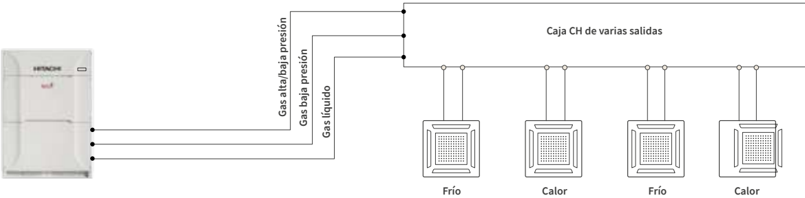
Caja CH de varias salidas: conexión en 3 tubos
