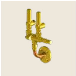
Doble válvula de seguridad Para proteger el circuito frigorífico de las altas presiones. De fábrica viene instalada una válvula simple. La válvula doble permite cambiar a una segunda válvula sin necesidad de vaciar el circuito frigorífico para las operaciones de mantenimiento. Ref.: DSV
