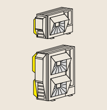
Campana de protección anti nieve trasera de acero inoxidable Ref. RAS-(2.0-3.0)WHVRP1 y RASM-(2-3)VRE: - ASG-SP10BTBS (semi) - Precio: 330 € Ref. RAS-(4.0-10.0)WH(V)NPE y RASM-(3-6)(V)NE: - ASG-NP280BS4 (semi) Precio: 550 € - ASG-SP11BAS2 (completa) Precio: 625 €
