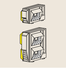
Campana de protección anti nieve trasera de zinc Ref. RAS-(2.0-3.0)WHVRP1 y RASM-(2-3)VRE: - ASG-SP10BTB Precio: 450 € Ref. RAS-(4.0-10.0)WH(V)NPE y RASM-(3-6)(V)NE: - ASG-NP160B (semi) Precio: 650 € - ASG-SP11BA (completa) Precio: 700 €
