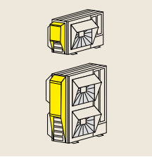
Campana de protección anti nieve izquierda de zinc Ref. RAS-(2.0-3.0)WHVRP1 y RASM-(2-3)VRE: - ASG-SP10LTB Precio: 330 € Ref. RAS-(4.0-10.0)WH(V)NPE y RASM-(3-6)(V)NE: - ASG-NP160L (semi) Precio: 370 € - ASG-SP11LA (completa) Precio: 400 €
