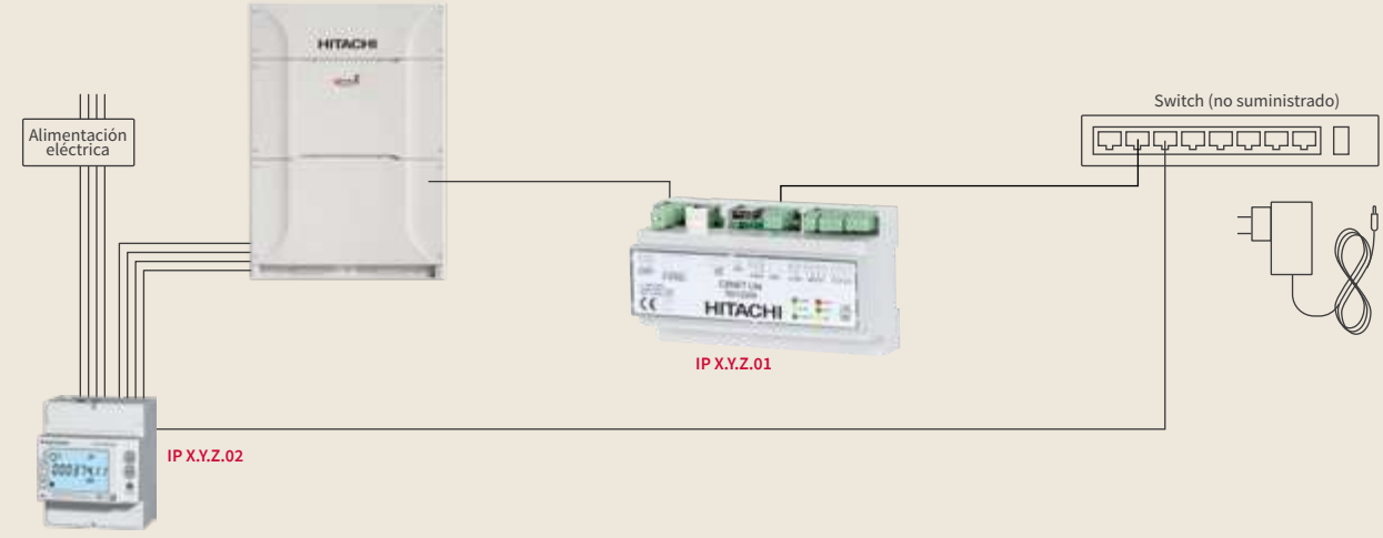
Caso de instalación con un circuito frigorífico y medidor de energía Ejemplo con un CSNET Lite
