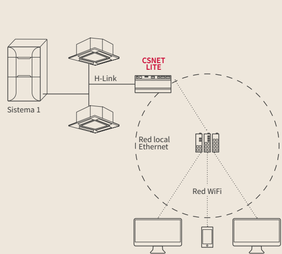
Ejemplo del cableado de una instalación pequeña (< 64 unidades interiores)
